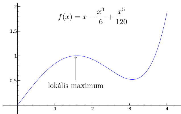
3. ábra. Függvény
