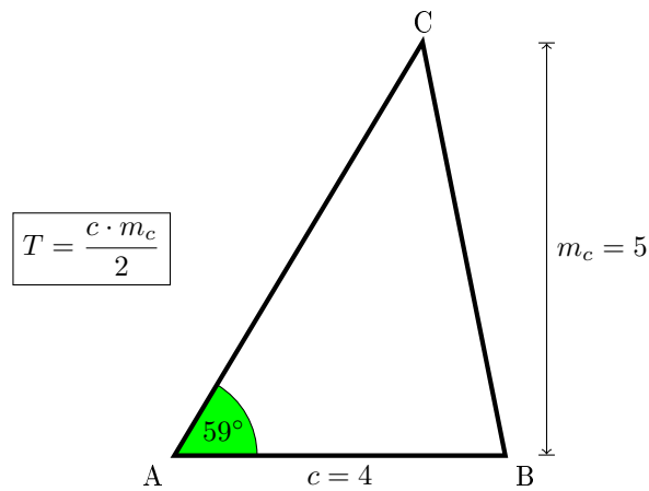
1. ábra. Háromszög
