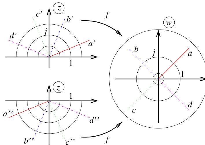
4.2. ábra. Az f(z) = z^2 kétrétű leképezés az origóból kiinduló, felső félsíkon levő a', b', c', d' illetve az alsó félsíkon levő a'', b'', c'', d'' félegyeneseket a képsík a, b, c, d félegyenesesire képezi. A leképezés a z félsíkokon berajzolt félköröket a w síkra berajzolt körökre képezi.
