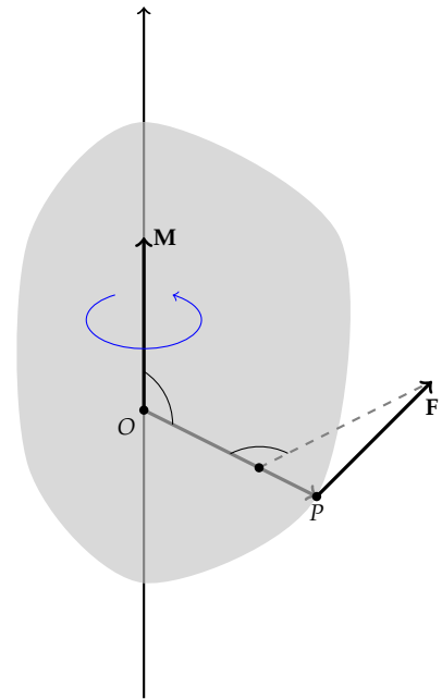
1.28. ábra: A test az O pontban rögzítve van, a P pontban hat az F erő, a forgás tengelye merőleges lesz az \vec{OP} és az F vektorok síkjára, az \vec{OP} , az F és \vec{M} jobbrendszert alkotnak, ahol \vec{M} a forgatónyomaték, melynek iránya megadja a forgatás irányát. Az |\vec{F}| \sin(\vec{OP}, \vec{F})_\angle szakaszt szaggatott vonal jelöli.
