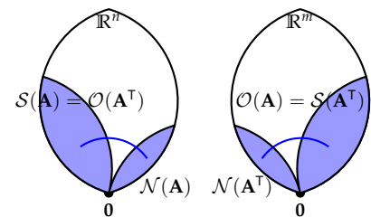
3.12. ábra: Az \mathbf{A} mátrix sortere merőleges nullterére, oszloptere az \mathbf{A}^\top nullterére. A berajzolt két ív az alterek merőlegességét jelöli.
