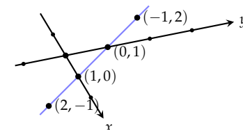
2.1. ábra: Az x + y = 1 egyenletet kielégítő néhány pont két különböző koordináta-rendszerben.
