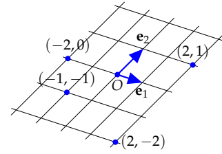
1.35. ábra: Pontok és koordinátáik
