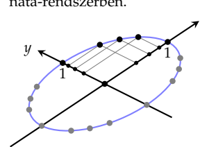
2.1. ábra: Az x + y = 1 egyenletet kielégítő néhány pont két különböző koordináta-rendszerben.
