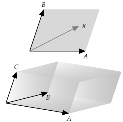
1.23. ábra: A paralelogramma és a paralelepipedon olyan lineáris kombinációkkal állítható elő, ahol az együtthatók 0 és 1 közé esnek.
