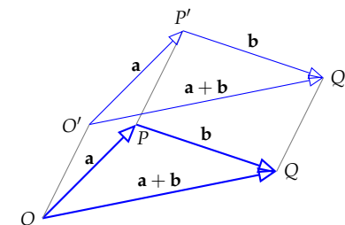
1.8. ábra: Az összeg független az O pont megválasztásától, ugyanis \vec{OQ} és \vec{O'Q'} azonos vektort reprezentál.
