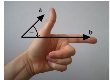
1.26. ábra: Két vektor egymáshoz való viszonya jobbrendszert (felső ábra) vagy balrendszert (alsó ábra) alkot. A közbe zárt irányított szög az előbbi esetben pozitív, utóbbiban negatív.
