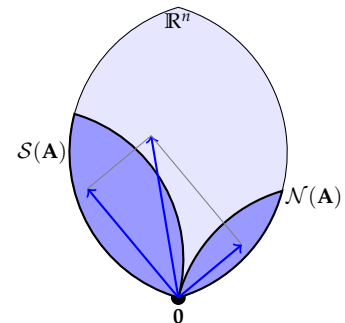
3.13. ábra: A lineáris algebra alaptétele: az \mathbf{A} mátrix sortere és nulltere merőleges kiegészítő alterek. Eszerint a sortér bármely vektora merőleges a nulltér bármely vektorára, és \mathbb{R}^n bármely vektora egyértelműen felbomlik egy sortérbe és egy nulltérbe eső vektor összegére.
