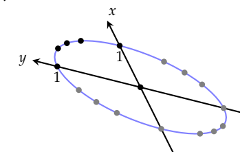
2.2. ábra: Az x^2 + y^2 = 1 egyenletet kielégítő (x, y) pontok halmaza két koordináta-rendszerben.
