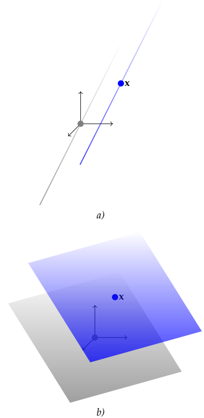
3.7. ábra: a) Egy háromismeretlenes inhomogén lineáris egyenletrendszer megoldáshalmaza, ha az általános megoldás egyparaméteres; b) Egy háromismeretlenes inhomogén lineáris egyenletrendszer megoldáshalmaza, ha az általános megoldás kétparaméteres.
