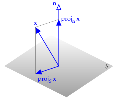
7.11. ábra: Vektor vetülete egy síkra
