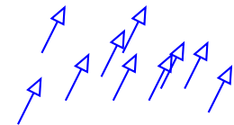
1.3. ábra: Ugyanazt a vektort reprezentáló irányított szakaszok
