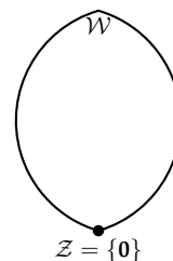
3.3. ábra: A \mathcal{W} vektortér két triviális altére: maga \mathcal{W} , és a \mathcal{Z} zérustér
