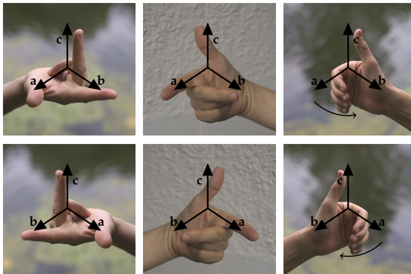
1.27. ábra: Az \mathbf{a} , \mathbf{b} és \mathbf{c} vektorok ebben a sorrendben jobbrendszert alkotnak, ha irányuk a jobb kezünkkel mutatható a mellékelt három ábra bármelyike szerint: (1) hüvelyk-mutató-középső ujj, (2) mutató-középső-hüvelykujj, (3) a hüvelyk mutatja a \mathbf{c} vektort, ökölbe szoruló kezünk ujjai pedig az \mathbf{a} felől a \mathbf{b} felé haladnak.
