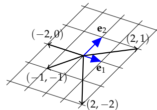
1.34. ábra: A megoldás helyvektorokkal ábrázolva.
