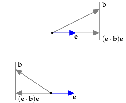
1.24. ábra: Az \mathbf{b} vektor és az \mathbf{e} egységvektor egyenesére eső vetülete. A felső ábrán \mathbf{e} \cdot \mathbf{b} > 0 , az alsón \mathbf{e} \cdot \mathbf{b} < 0 .
