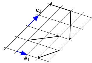
1.32. ábra: Mik a vektorok koordinátái? (-2, 0)
