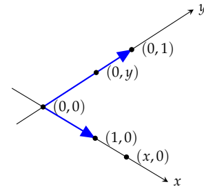
1.36. ábra: Pontok a koordináta-rendszer tengelyein.
