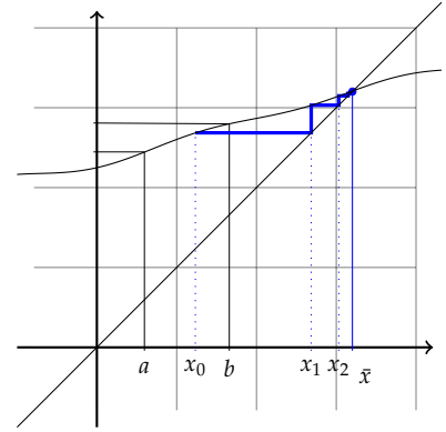
2.13. ábra: Egy függvény, mely bármely a és b pontot két olyan pontba visz, melyek távolsága a és b távolságának legföljebb a fele, így a függvény minden különbségi hányadosa abszolút értékben legföljebb 1/2 . E függvénynek pontosan egy fixpontja van, mely megkapható egy tetszőleges x_0 pontból induló x_k = f(x_{k-1}) sorozat határértékeként.
