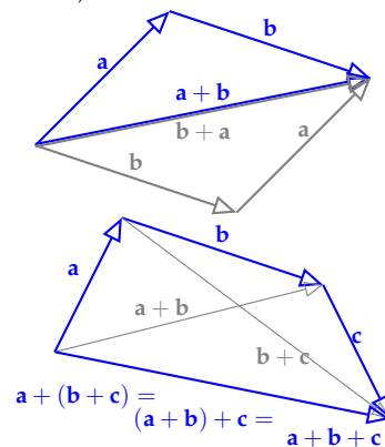
1.11. ábra: A vektorösszeadás kommutativitása és asszociativitása.
