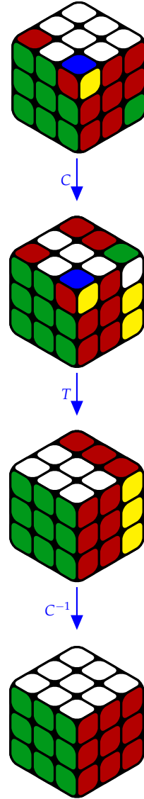
7.17. ábra: A felső kockán látható három csúcskockát kell kicserélni. Először a három csúcst egy síkba mozgatjuk ( \mathbf{C} transzformáció), majd az előző ábrán látható \mathbf{T} transzformációval kicseréljük őket, végül \mathbf{C} inverzének alkalmazása után minden kocka a helyére kerül. Így a transzformációk egymás utáni elvégzését szorzásnak tekintve a megoldást a \mathbf{C} \mathbf{T} \mathbf{C}^{-1} transzformáció adja.
