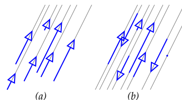
1.5. ábra: (a) egyirányú vektorok, (b) kollineáris (párhuzamos) vektorok, vannak köztük egyirányúak és ellenkező irányúak
