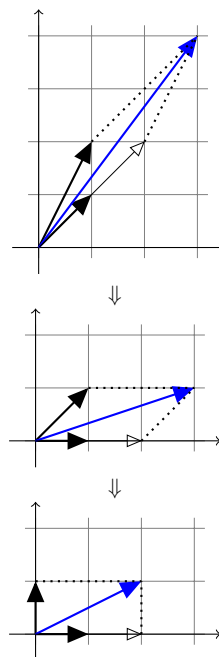
2.10. ábra: A megoldás lépései a oszlopmodellben.
