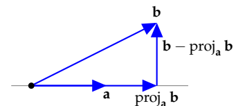
1.25. ábra: Az \mathbf{b} vektor felbontása az \mathbf{a} vektorral párhuzamos és rá merőleges vektorok összegére.
