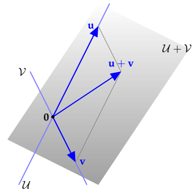
7.19. ábra: \mathcal{U} + \mathcal{V} bármely vektora előáll \mathbf{u} + \mathbf{v} alakban
