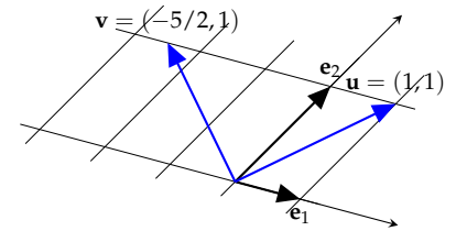
1.38. ábra: Két vektor skaláris szorzata
