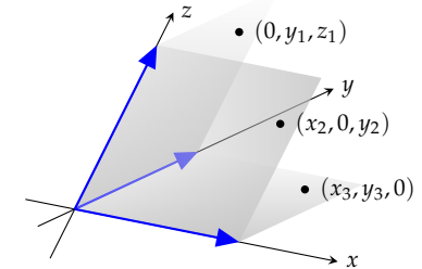
1.37. ábra: Pontok a koordinátasíkokon
