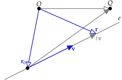
2.3. ábra: Egyenes explicit vektoregyenlete: \mathbf{r} = \mathbf{r}_0 + t\mathbf{v} .
