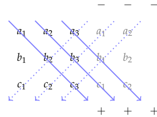
1.41. ábra: A paralelepipedon térfogata megegyezik az azt kifeszítő három vektor vegyes szorzatának abszolút értékével. A vektori szorzáshoz használt séma itt is működik: a három vektort egymás alá írjuk, az így kapott táblázat első két oszlopát utána másoljuk, végül a \searrow nyíl menti szorzatokból kivonjuk a \swarrow menti szorzatokat. A később tanulandó determinánsokra használt jelöléssel tehát a paralelepipedon előjeles térfogata:
