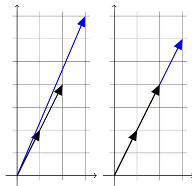
2.11. ábra: Oszlopmodell lineárisan összefüggő vektorok esetén.
