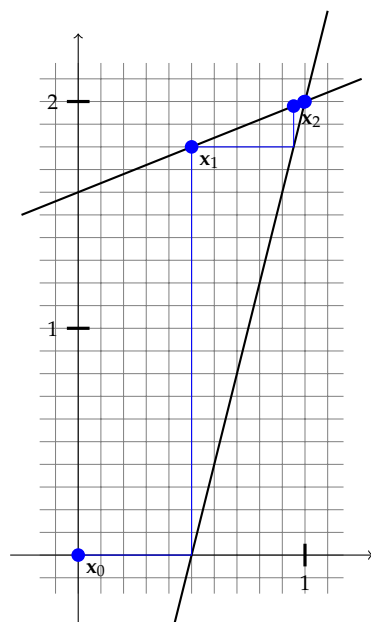
2.15. ábra: A Gauss–Seidel-iteráció szemléltetése
