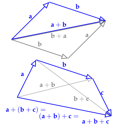
1.11. ábra: A vektorösszeadás kommutativitása és asszociativitása.
