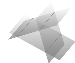
(b) Egy egyenessel párhuzamos, de közös egyenest nem tartalmazó három sík 2.9. ábra: Nem megoldható egyenletrendszerek
