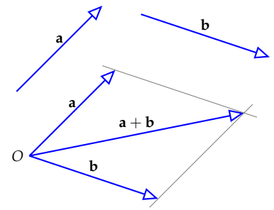
1.9. ábra: Parallelogramma-módszer
