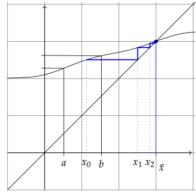
2.13. ábra: Egy függvény, mely bármely a és b pontot két olyan pontba visz, melyek távolsága a és b távolságának legföljebb a fele, így a függvény minden különbségi hányadosa abszolút értékben legföljebb 1/2 . E függvénynek pontosan egy fixpontja van, mely megkapható egy tetszőleges x_0 pontból induló x_k = f(x_{k-1}) sorozat határértékeként.
