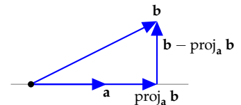
1.26. ábra: Az \mathbf{b} vektor felbontása az \mathbf{a} vektorral párhuzamos és rá merőleges vektorok összegére.
