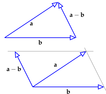
1.12. ábra: A különbségvektor meghatározása háromszög- és parallelogrammamódszerrel.
