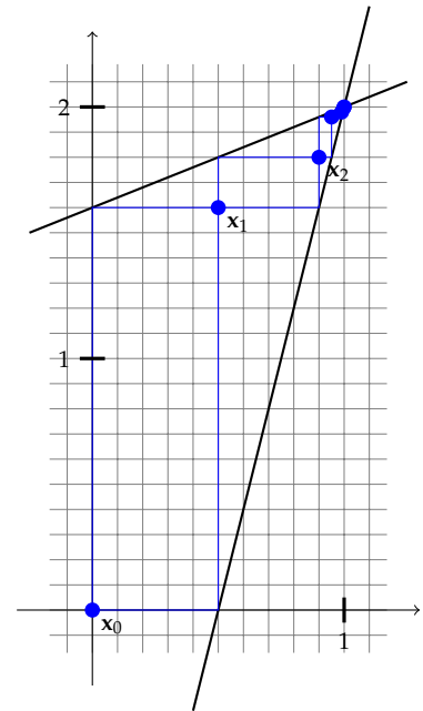
2.14. ábra: A Jacobi-iteráció szemléltetése
