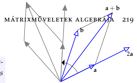
5.4. ábra: A pont körüli elforgatás lineáris leképezés
