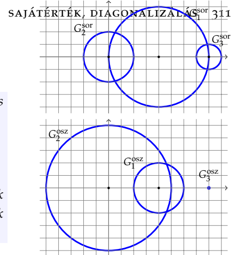
8.3. ábra: Az \mathbf{A} mátrix Gerschgorin körei
