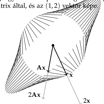
5.10. ábra: Az A = \begin{bmatrix} 5/4 & 3/4 \\ 3/4 & 5/4 \end{bmatrix} mátrix hatását szemlélteti oly módon, hogy az egységkör néhány pontját összeköti a képükkel. Az ábrán egy egységnyi x vektort és Ax képét, valamint a 2x vektort és képét a A(2x) = 2Ax vektort kiemeltük.
