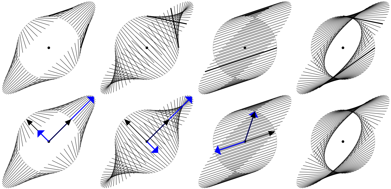
5.12. ábra: Négy leképezés egységkör-ábrája a bázisvektorokat és képüket összekötő vonalak kiemelésével, és a saját maguk konstansszorosába képzett vektorokkal.
