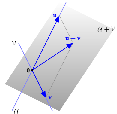
3.7. ábra: \mathcal{U} + \mathcal{V} bármely vektora előáll \mathbf{u} + \mathbf{v} alakban
