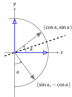
6.12. ábra: Az \mathbf{i} és \mathbf{j} vektorok egy egyenesre való tükröképe
