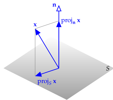
6.11. ábra: Vektor vetülete egy síkra
