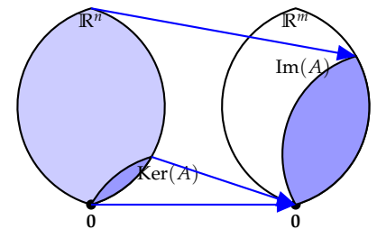
5.13. ábra: Egy A : \mathbb{R}^n \rightarrow \mathbb{R}^m, x \mapsto Ax mátrixleképezés levéldiagramja. Az ábrán három altér színezéssel ki van emelve – az értelmezési tartomány ( \mathbb{R}^n ), az értékkészlet ( \text{Im}(A) = \mathcal{O}(A) ) és a magtér ( \text{Ker}(A) = \mathcal{N}(A) ).
