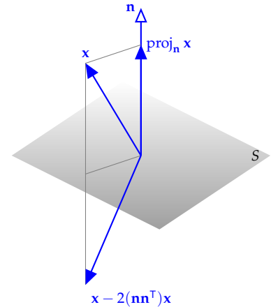
6.13. ábra: Vektor tükröképe egy síkra
