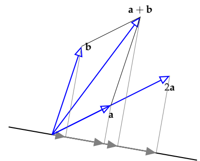
5.6. ábra: Az egyenesre való merőleges vetítés lineáris leképezés
