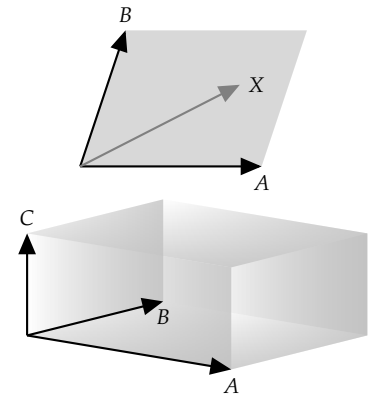
1.23. ábra: A parallelogramma és a parallelepipedon olyan lineáris kombinációkkal állítható elő, ahol az együtthatók nem negatívak, és összegük legfeljebb 1.
