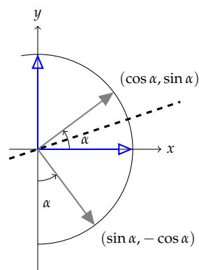
7.20. ábra: Az \mathbf{i} és \mathbf{j} vektorok egy egyenesre való tükörképe
