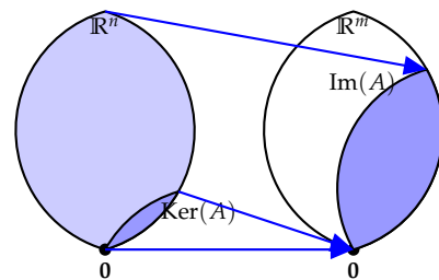
7.7. ábra: Egy A : \mathbb{R}^n \rightarrow \mathbb{R}^m, \mathbf{x} \mapsto \mathbf{A}\mathbf{x} mátrixleképezés levéldiagrammja. Az ábrán három altér színezéssel ki van emelve – az értelmezési tartomány ( \mathbb{R}^n ), az értékkészlet ( \text{Im}(A) = \mathcal{O}(\mathbf{A}) ) és a magtér ( \text{Ker}(A) = \mathcal{N}(\mathbf{A}) ).
