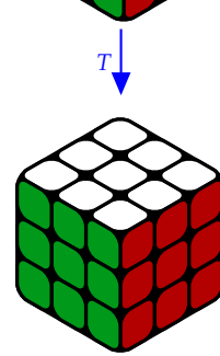
7.13. ábra: A T transzformáció a bűvös kocka egy lapon lévő 3 csúcsát ciklikusan fölcseréli egymással (a jobb felsőt sarokban lévő a bal sarokba, azt a középsőbe viszi), az összes többi helyben hagyja. Mit tegyünk ha 3 nem egy lapon lévő csúcsot kell ciklikusan fölcserélni?
