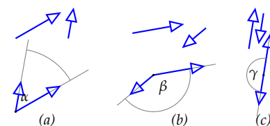
1.6. ábra: Két vektor szöge ( 0 \leq \alpha, \beta, \gamma \leq \pi ). Az ábra felső felén a két adott vektor, alatta szögük meghatározásának módja szerepel.
