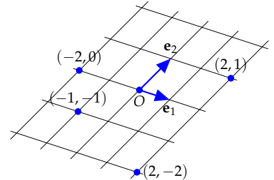
1.36. ábra: Pontok és koordinátáik
