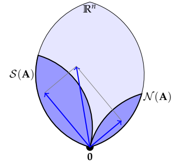
3.14. ábra: A lineáris algebra alaptétele: az \mathbf{A} mátrix sortere és nulltere merőleges kiegészítő alterek. Eszerint a sortér bármely vektorára, és \mathbb{R}^n bármely vektora egyértelműen felbomlik egy sortérbe és egy nulltérbe eső vektor összegére.
