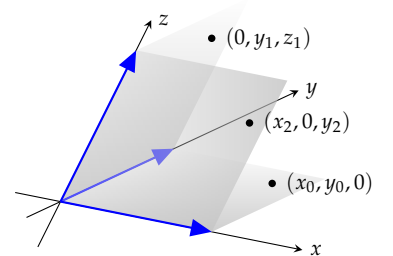
1.38. ábra: Pontok a koordinátasíkokon
