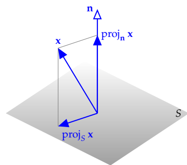
7.19. ábra: Vektor vetülete egy síkra
