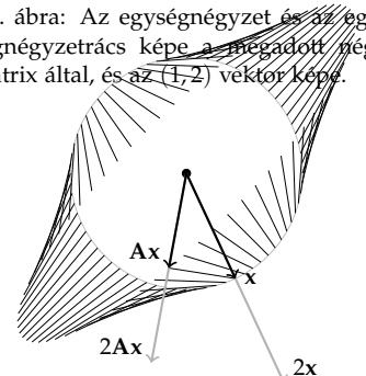
7.4. ábra: Az A = \begin{bmatrix} 5/4 & 3/4 \\ 3/4 & 5/4 \end{bmatrix} mátrix hatását szemlélteti oly módon, hogy az egységkör néhány pontját összeköti a képükkel. Az ábrán egy egységnyi x vektort és Ax képét, valamint a 2x vektort és képét a A(2x) = 2Ax vektort kiemeltük.
