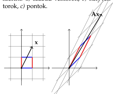
7.2. ábra: Az \mathbf{A} = \begin{bmatrix} 1 & 1 \\ 1 & 2 \end{bmatrix} mátrix hatása az egységnégyzetrácsra, és az \mathbf{x} = (1, 2) vektoron. Az \mathbf{Ax} vektor végpontja a paralelogrammarácsra 1 lépés az x -tengely képének irányába, és 2 lépés az y -tengely képének irányába.
