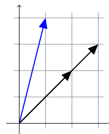
2.11. ábra: Tekintsük a nyilvánvalóan ellentmondó 2x + 3y = 1 , 2x + 3y = 4 egyenletrendszert, és annak oszlopmodell alakját: (2,2)x + (3,3)y = (1,4) . Mivel a (2,2) és a (3,3) vektorok lineáris kombinációjaként csak (c,c) alakú vektor állítható elő, az (1,4) vektor nem, ezért a fenti egyenletrendszernek nincs megoldása.
