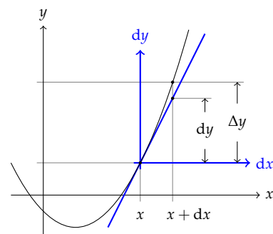
7.15. ábra: A dx és dy koordinátatengelyeket és a dy = Ddx függvény grafikonját színezéssel kiemeltük. Az ábra egyúttal a \Delta y \approx dy kapcsolatot is szemlélteti.
