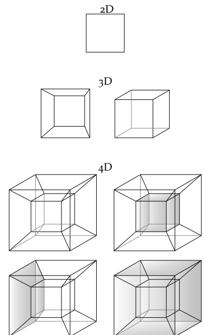
1.40. ábra: 4-dimenziós kocka ábrázolása 2-dimenzióban.
