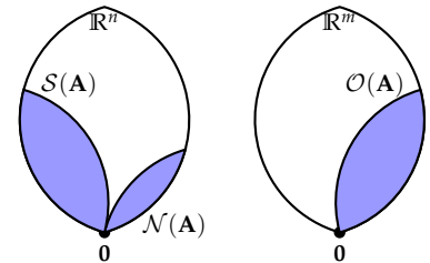
3.10. ábra: Az \mathbf{A} mátrix sortere ( \mathcal{S}(\mathbf{A}) ), oszloptere ( \mathcal{O}(\mathbf{A}) ) és nulltere ( \mathcal{N}(\mathbf{A}) ).
