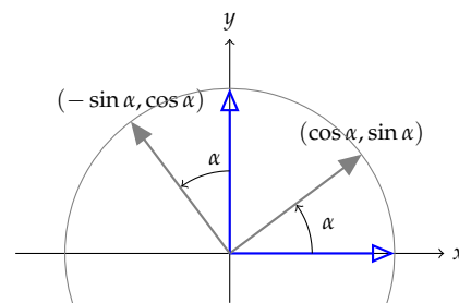
7.18. ábra: Az \mathbf{i} és \mathbf{j} vektorok \alpha szöggel való elforgatottjai
