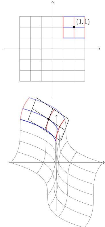
7.16. ábra: A felső ábra az \mathbf{f}(x, y) = (-x^3/2 + y^3/8, x + y) függvény értelmezési tartományán megadott rácsot, és annak egy kis 2 \times 2 -es részét mutatja, melynek középpontja az (1, 1) pont. Az alsó ábra egyrészt halványan jelöli e rács és színesen a kiemelt rács képét, valamint az (1, 1) ponthoz tartozó deriváltleképezés hatását e kiemelt rácson.
