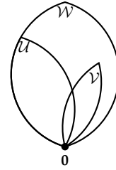
3.2. ábra: Egy \mathcal{W} vektortér és annak \mathcal{U} és \mathcal{V} alterei, valamint a mindannyiukban közös nullvektor
