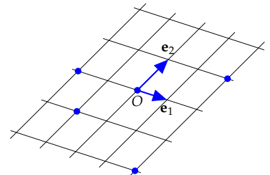
1.35. ábra: Mik a pontok koordinátái?
