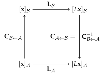
7.12. ábra: Ezt az ábrát az előzőből egyetlen nyíl és felírata megváltoztatásával kaptuk. Erről közvetlenül leolvasható az \mathbf{L}_\mathcal{A} = \mathbf{C}_{\mathcal{A} \leftarrow \mathcal{B}}\mathbf{L}_\mathcal{B}\mathbf{C}_{\mathcal{B} \leftarrow \mathcal{A}} , illetve az \mathbf{L}_\mathcal{A} = \mathbf{C}_{\mathcal{B} \leftarrow \mathcal{A}}^{-1}\mathbf{L}_\mathcal{B}\mathbf{C}_{\mathcal{B} \leftarrow \mathcal{A}} összefüggés. Ehhez az [\mathbf{x}]_\mathcal{A} -ból az [L\mathbf{x}]_\mathcal{A} -ba vezető két utat kell bejárunk, és közben a megfelelő mátrixokat összeszorozunk.
